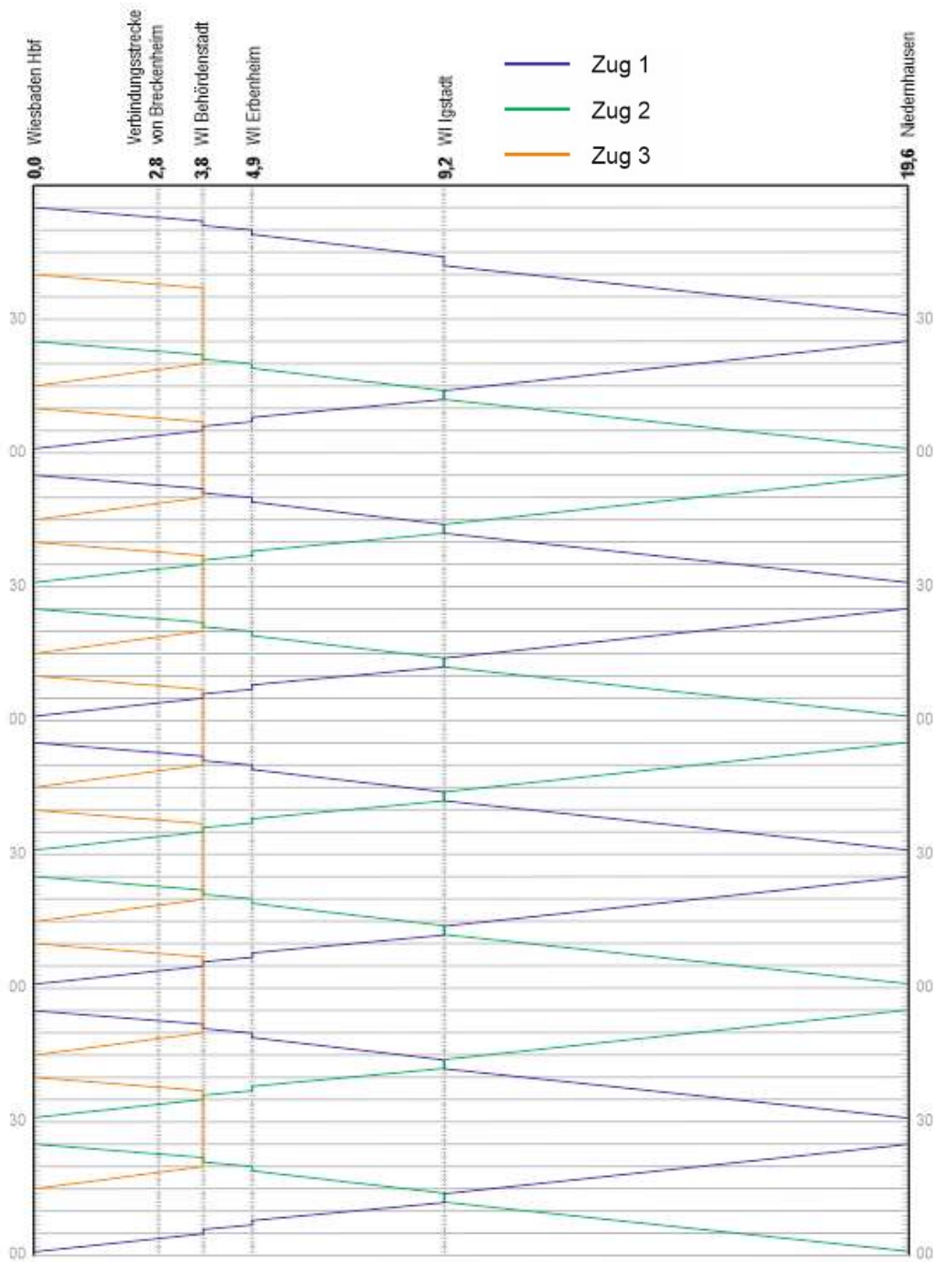
Abbildung 18: Zeit-Weg-Diagramm Ländchesbahn Vorzugsvariante (Planfall 1b)
