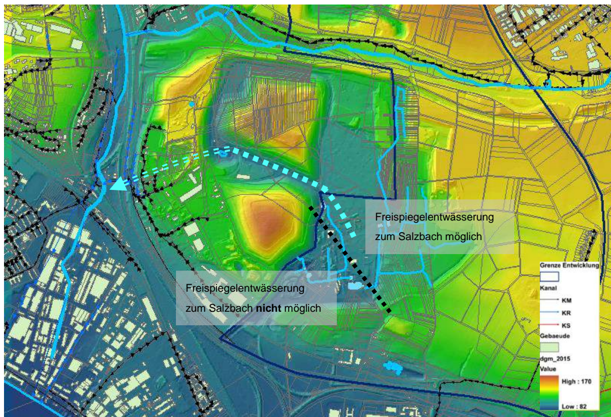
Abb. 3-8: Ableitungsmöglichkeiten für das Regenwasser in den Salzbach
