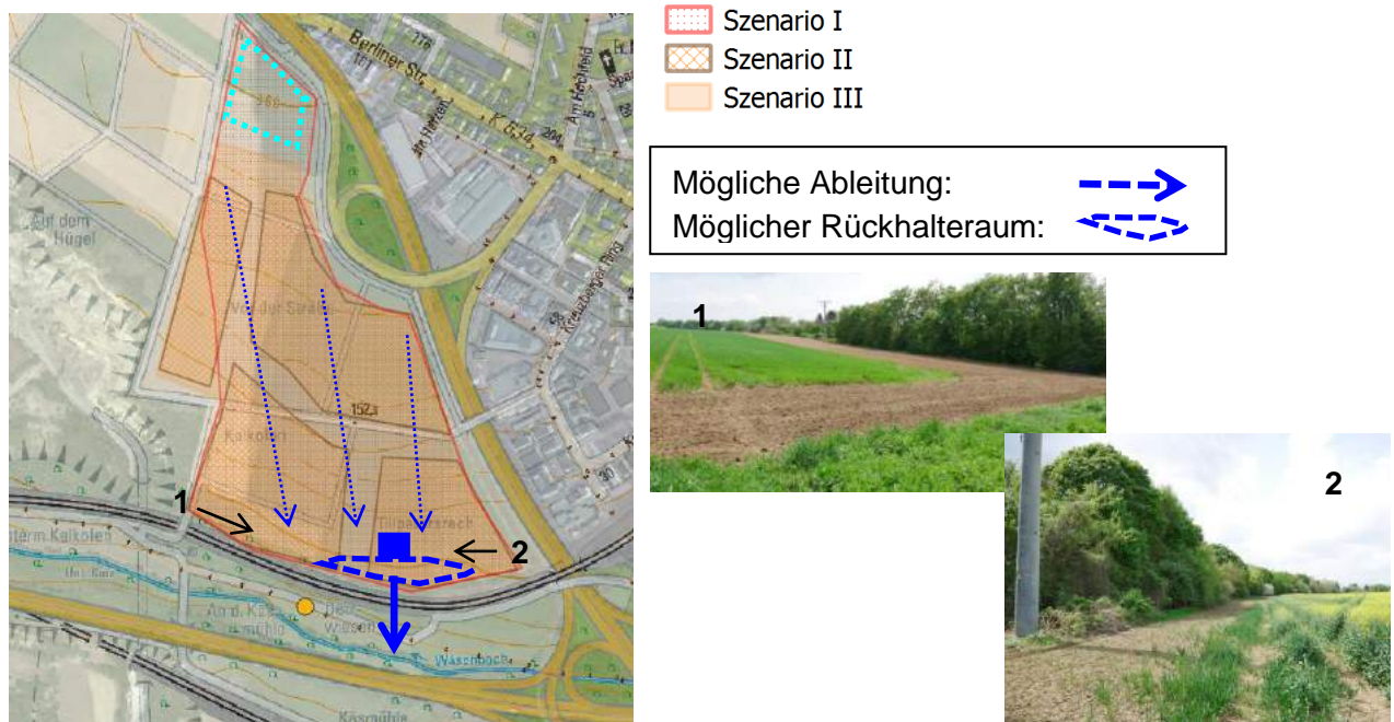
Abb. 6-2: Skizze Rückhalt und Ableitung in Wäschbach
